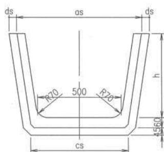
端面図
