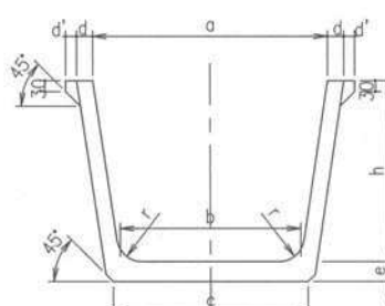
A-A断面図
