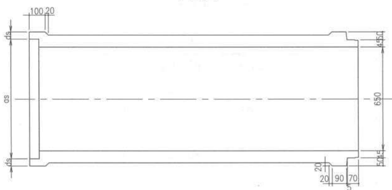
A-A断面図
