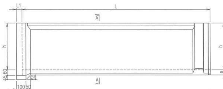
側面図
