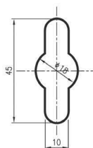
吊り金具詳細図
