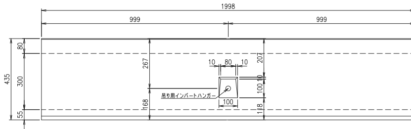
側面図
