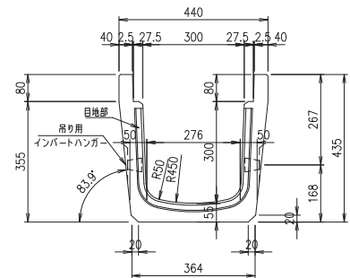
端面図
