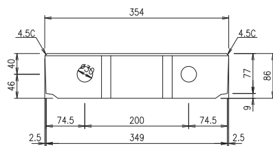
断面図
