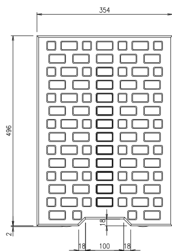
平面図
