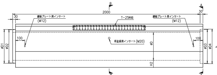
側面図
