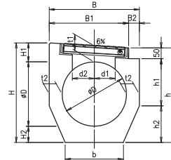
B ~ B 断面図
