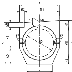
A ~ A 端面図
