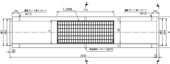
平面図
