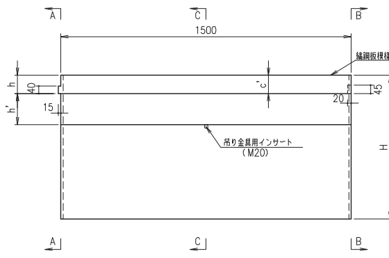
平面図
