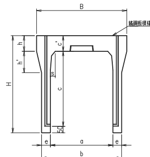
C～C 断面図
