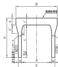
C～C 断面図
