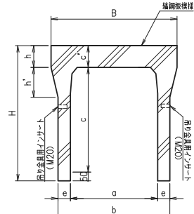
C～C 断面図
