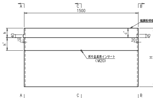
側面図
