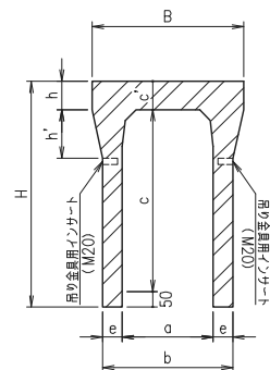
C～C 断面図
