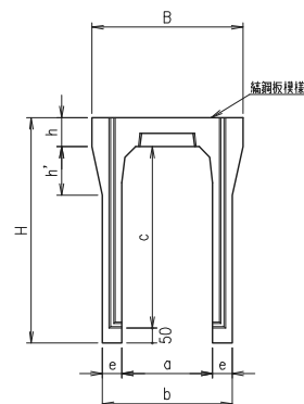
C～C 断面図
