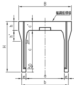
A～A 端面図
