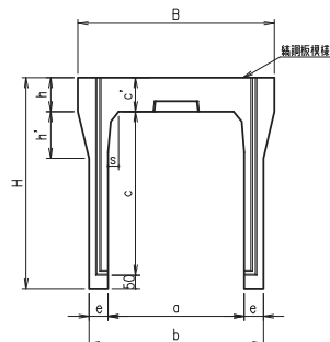
A～A 端面図
