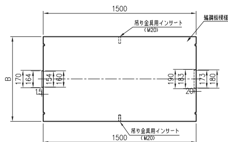
平面図
