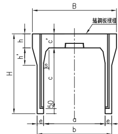
C～C 断面図
