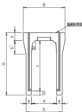
A～A 端面図
