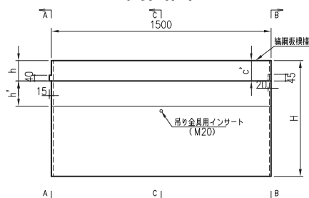
側面図
