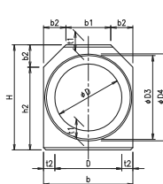
A～A 端面図
