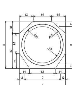
A～A 端面図
