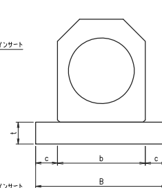
施工断面図
