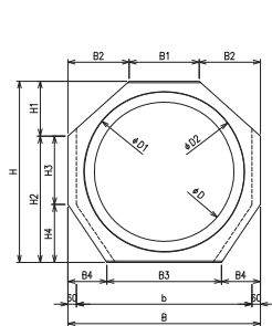
B～B 端面図
