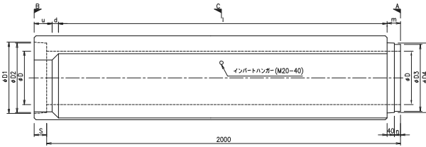
平面図
