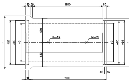
平面図
