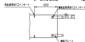
連結プレート詳細図
