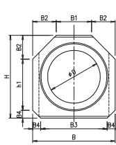
B～B 端面図
