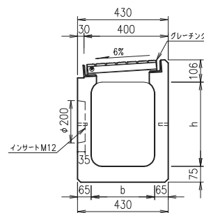
A～A断面図
