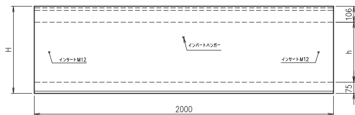
側面図
