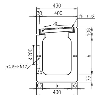
A～A 断面図
