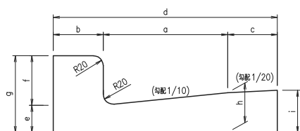
側面図
