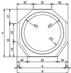
B ~ B 端面図
