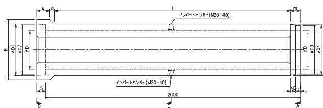
平面図
