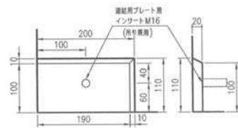
A 連結部詳細図
