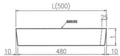
側面図
