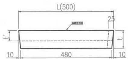
側面図
