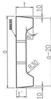
側面図
