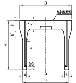
C～C 断面図
