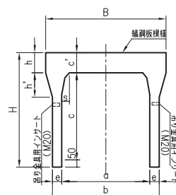
C～C 断面図
