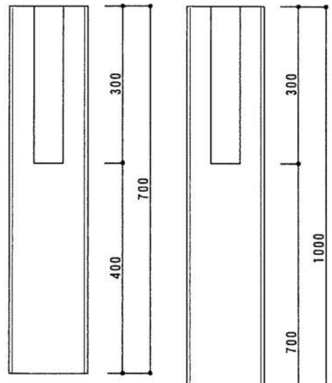
鉄管防護柱 L = 700 重量 34kg
