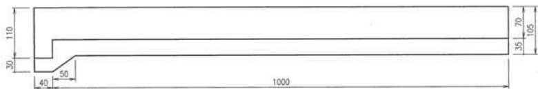
端面図
