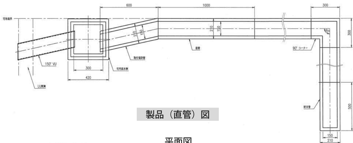
宅内雨水排水セット平面図
