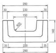
端面図
