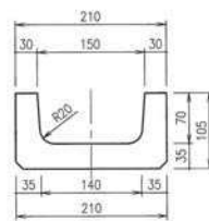
端面図
