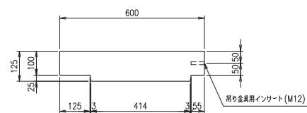
側面図
