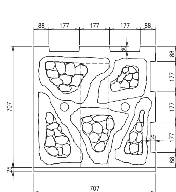
正面図
