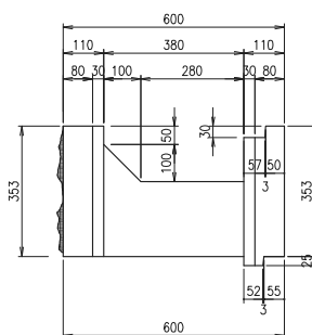
側面図
