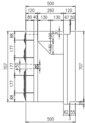
側面図
