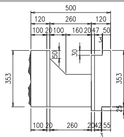
側面図
