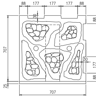
正面図
