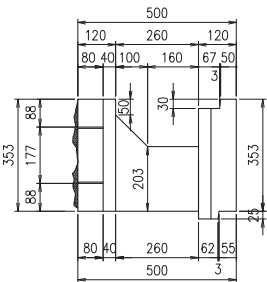
側面図
