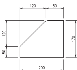
側面図
