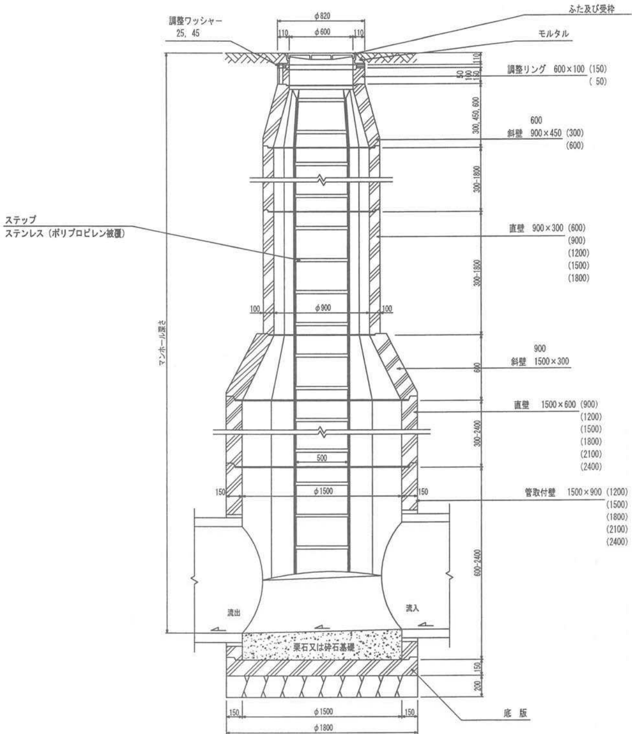
縦断面図
