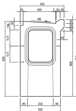
端面图
