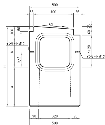
端面図
