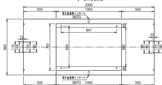
平面图
