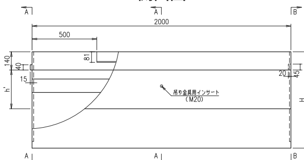
側面図
