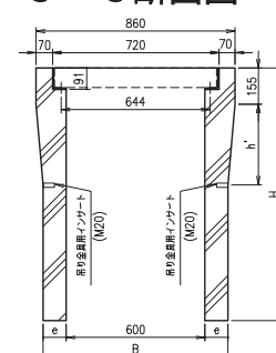
C~C断面図
