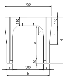
C～C 断面図
