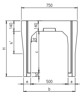
A～A 端面図
