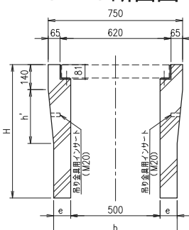
C～C 断面図
