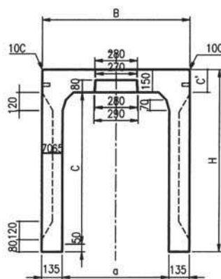
端面図
