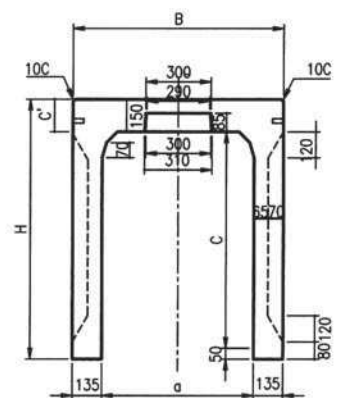
端面図
