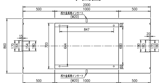
平面图
