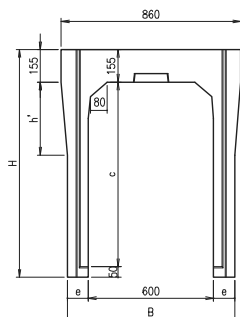
A ~ A 端面图
